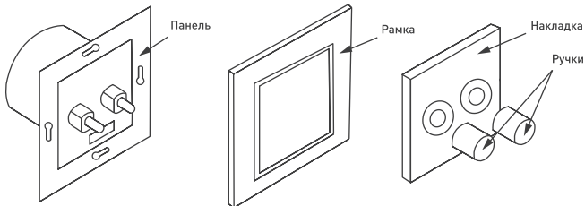
Рисунок 3. Установка декоративной накладкой для панели LN-100-DUAL (в комплект поставки не входит).
